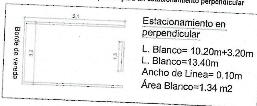
Fig. N° 05 – Metrado de pintura para un estacionamiento perpendicular
