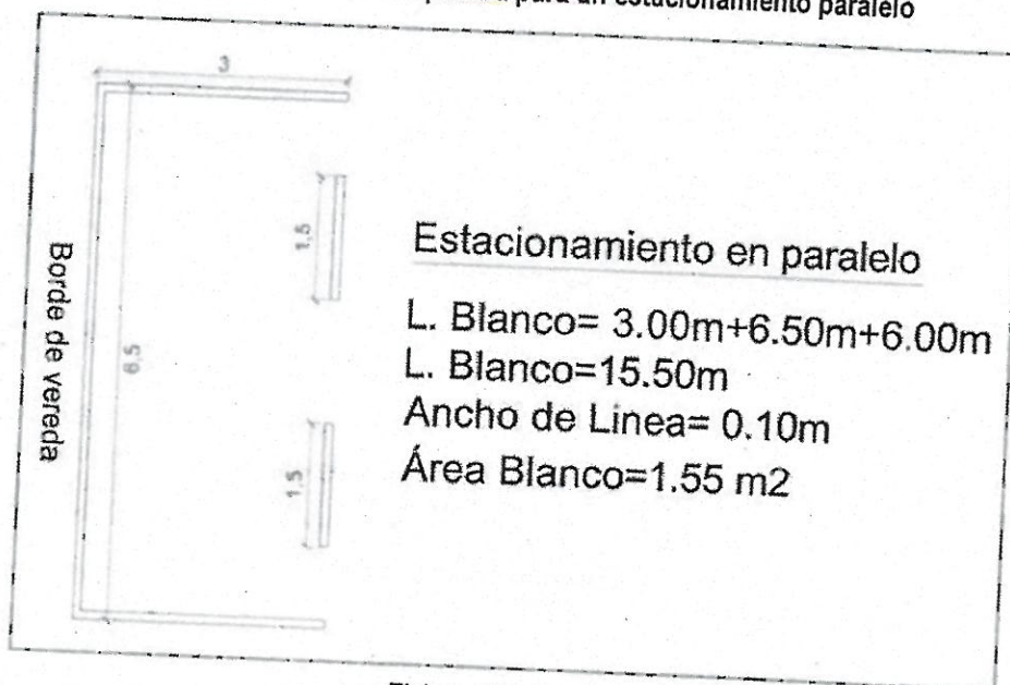
Fig. N° 04 – Metrado de pintura para un estacionamiento paralelo
